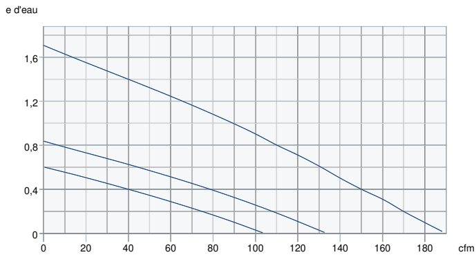
Soufflage - Courbe de performance
